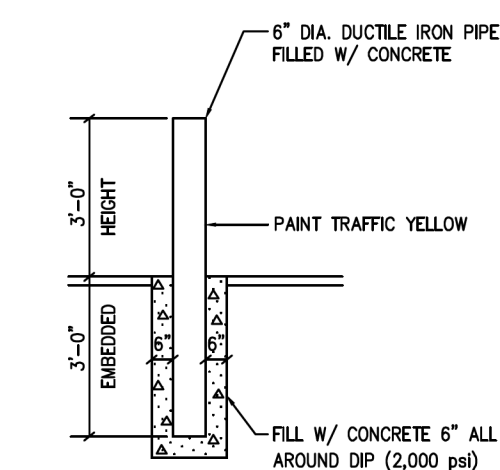
BOLLARD DETAIL N.T.S.
